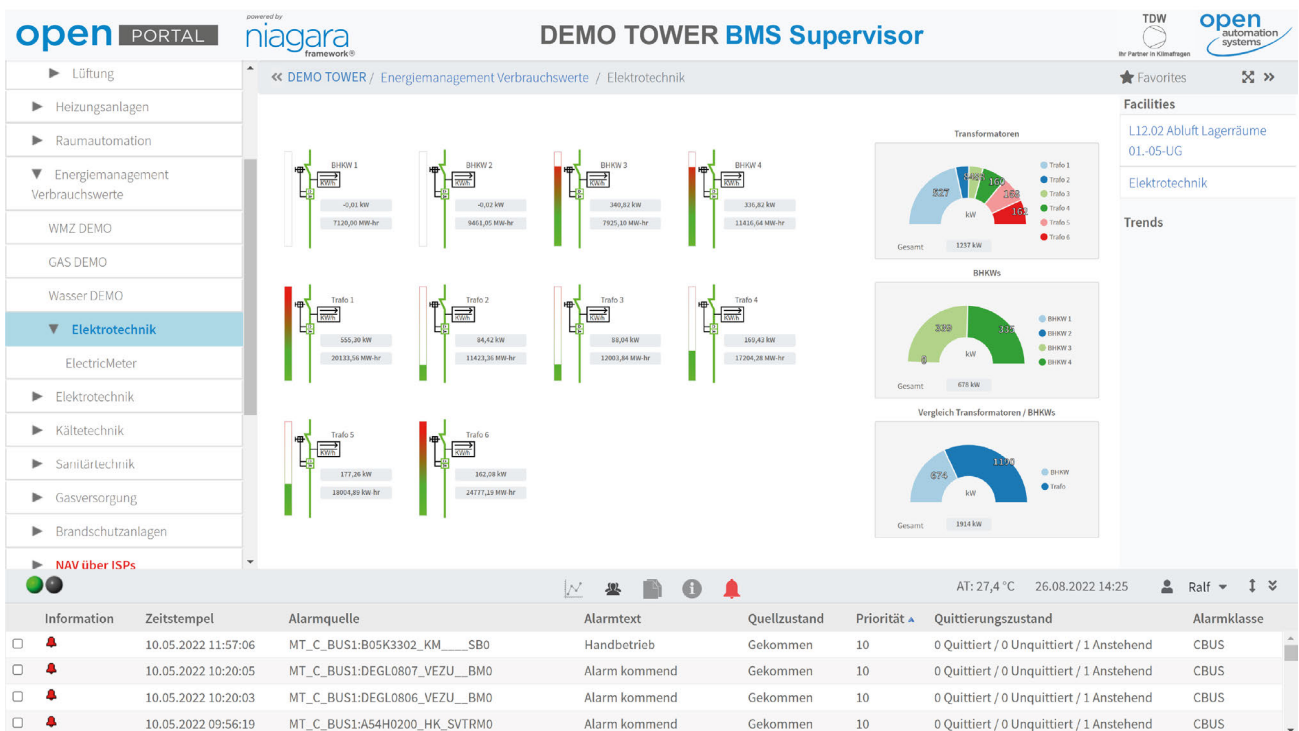
Beispiel der Darstellung des Energiemanagement-Dashboards für die Verbrauchswerte des Main Tower
